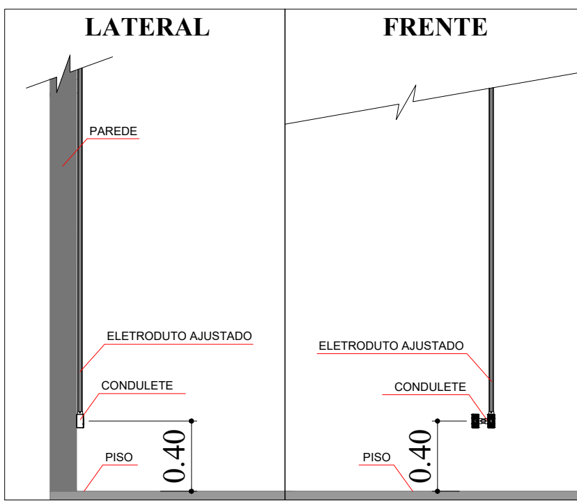
TOMADAS AJUSTADAS
