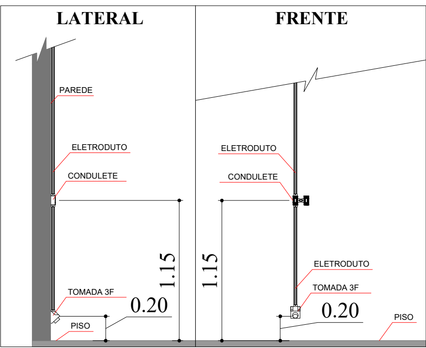
INTERRUPTORES / TOMADA EXISTENTE
