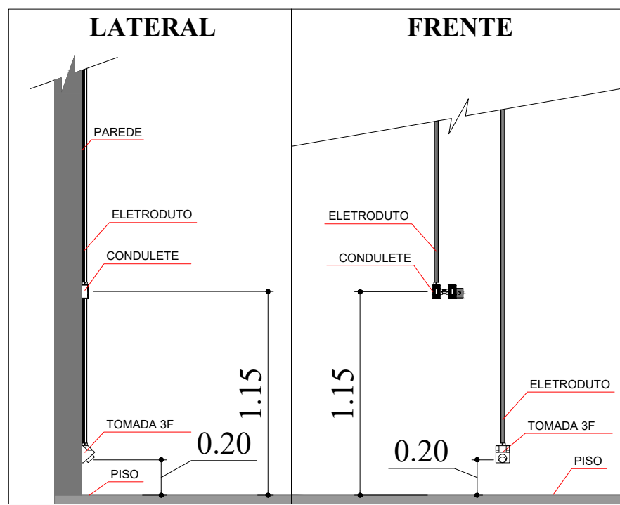
INTERRUPTORES EXISTENTE
