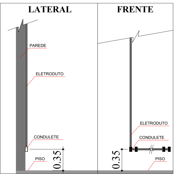
TOMADAS EXISTENTE
