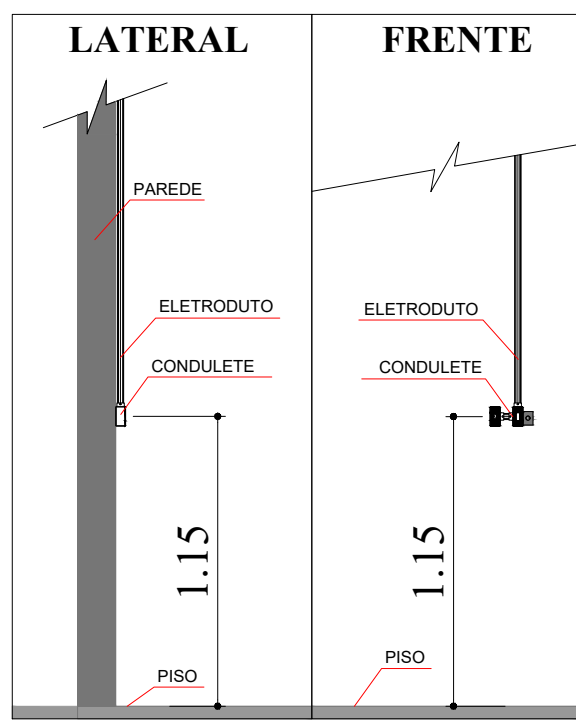
INTERRUPTOR / TOMADA EXISTENTE
