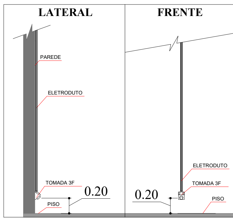
TOMADA EXISTENTE
