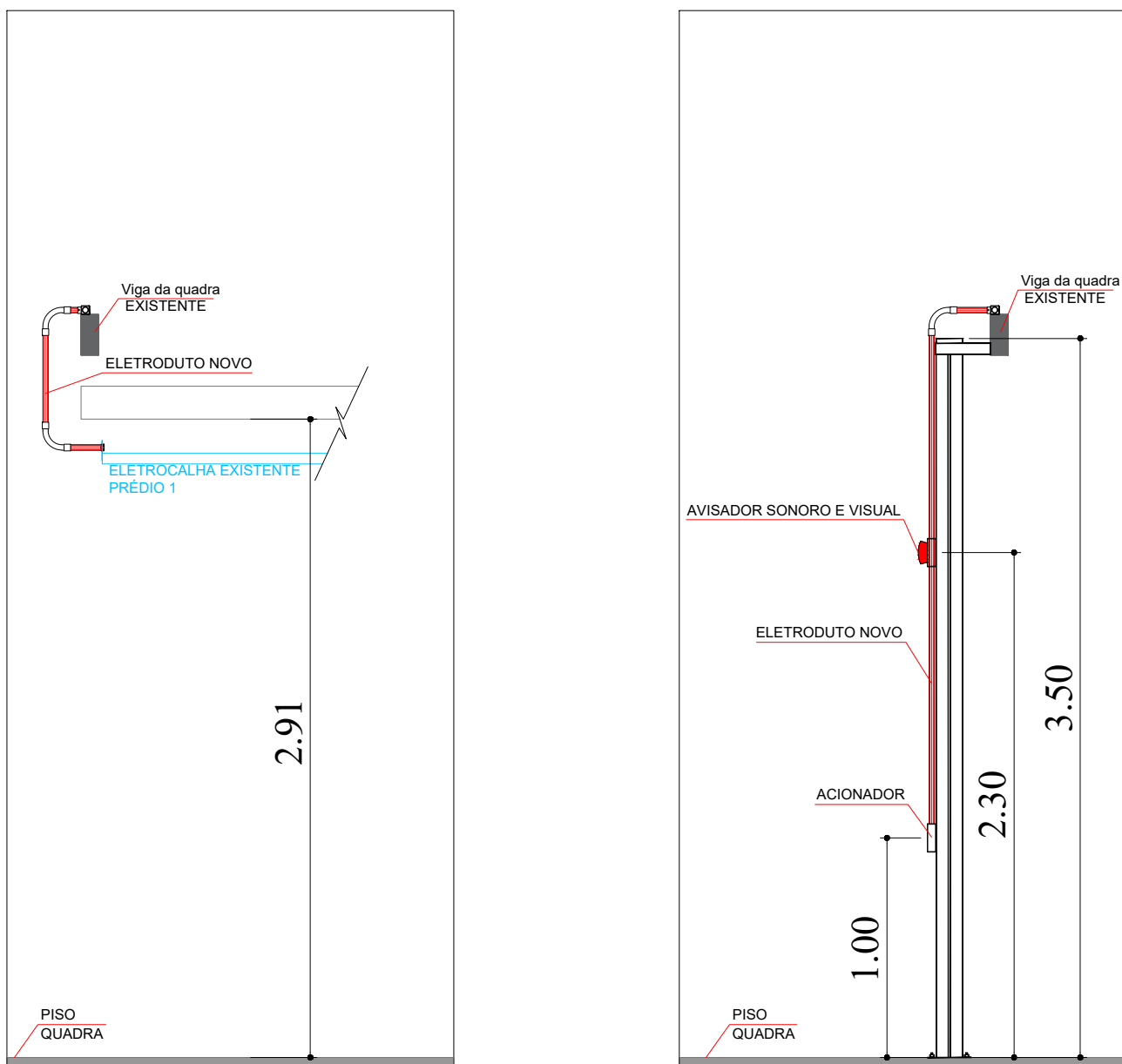
LIGAÇÃO DO PRÉDIO 01 COM A QUADRA
