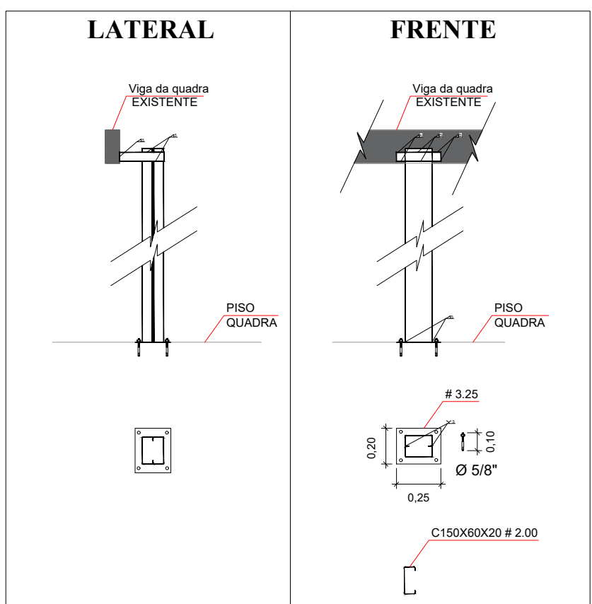
PILAR METÁLICO DE APOIO QUADRA POLIESPORTIVA
