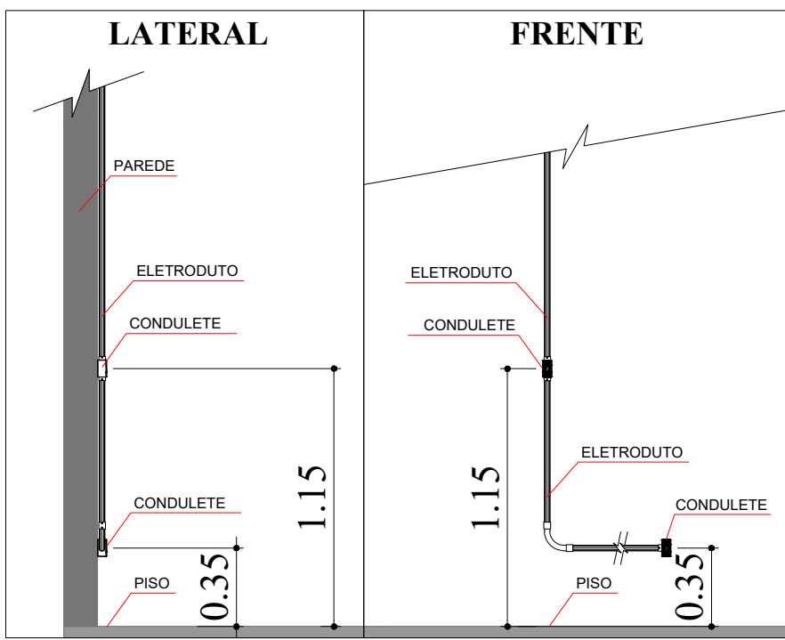
TOMADAS EXISTENTES
