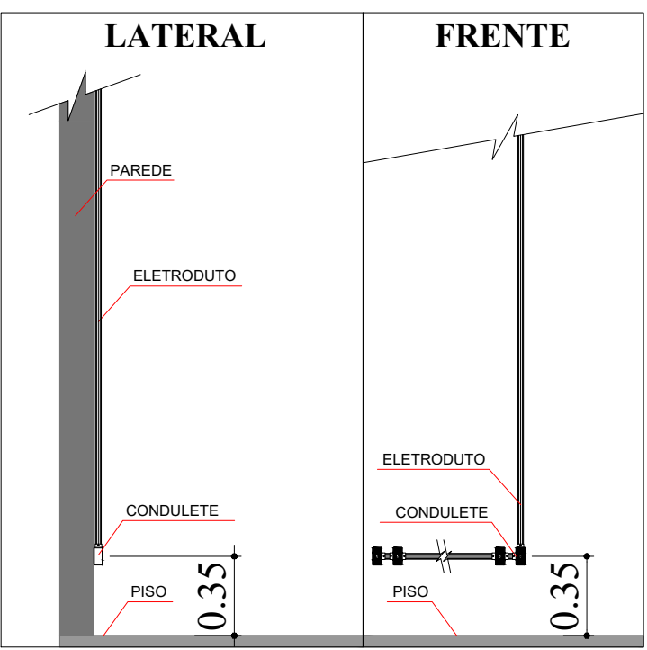
TOMADAS EXISTENTE
