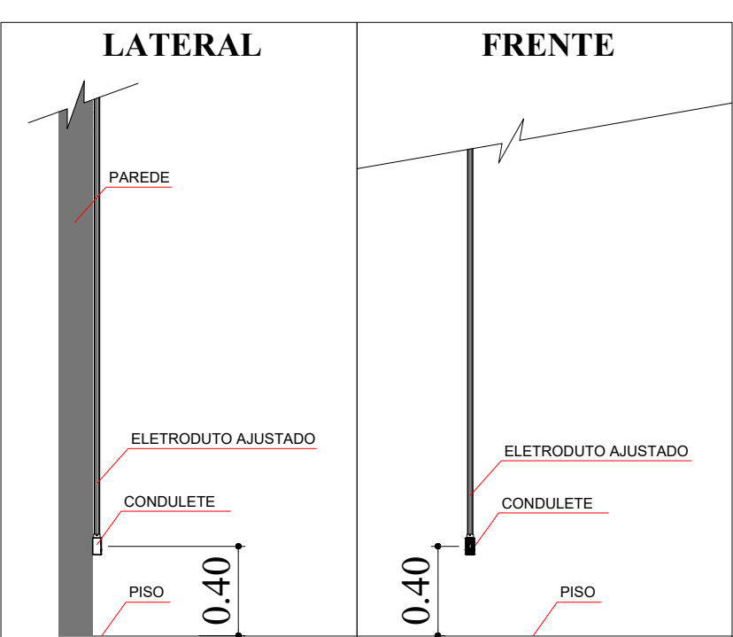
TOMADA AJUSTADA
