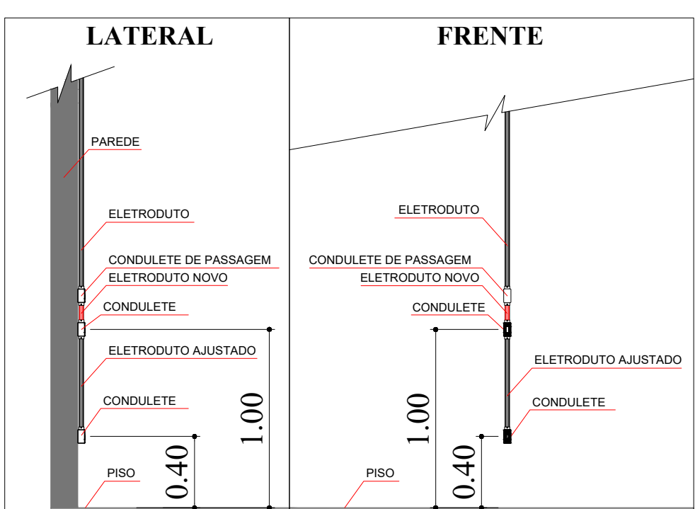
INTERRUPTOR / TOMADA AJUSTADOS
