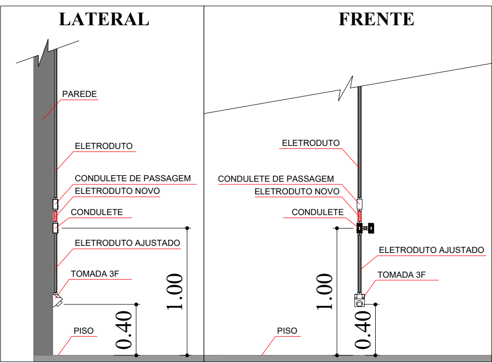
INTERRUPTORES / TOMADA AJUSTADOS
