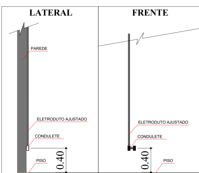
TOMADAS AJUSTADAS
