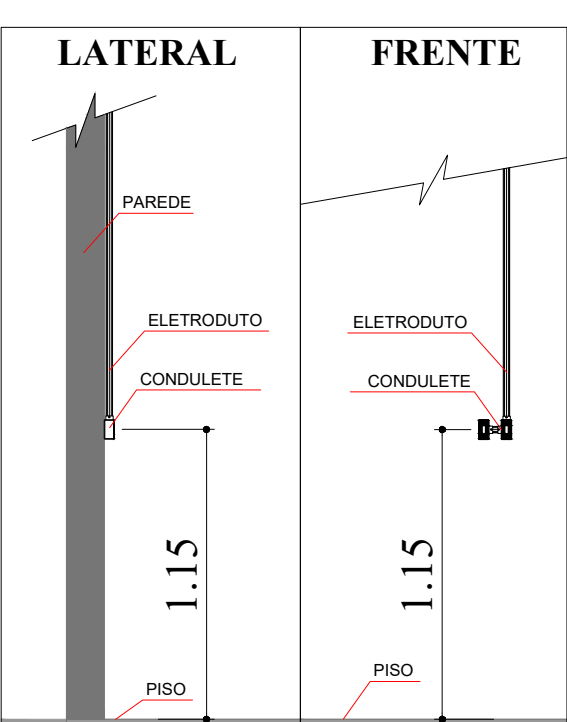
INTERRUPTORES EXISTENTES
