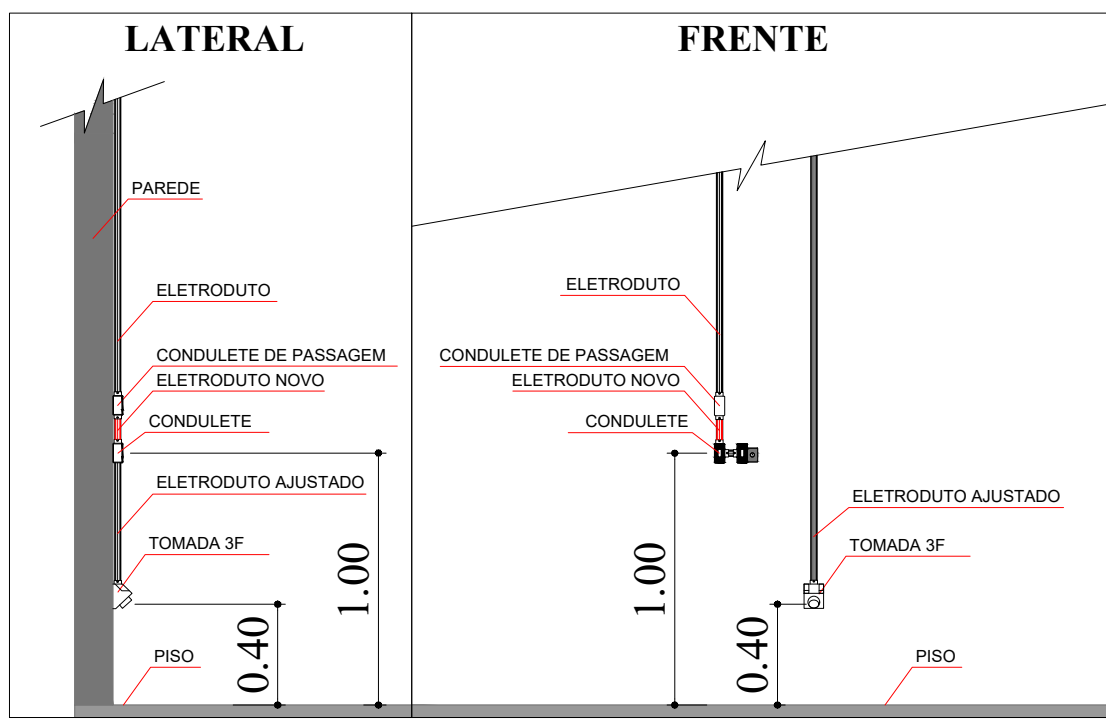
INTERRUPTORES AJUSTADOS
