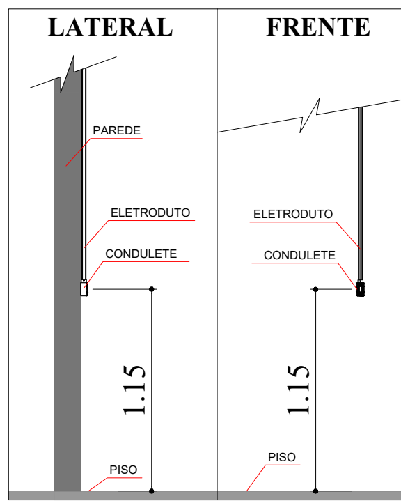
INTERRUPTOR EXISTENTE
