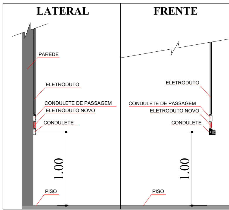
INTERRUPTOR AJUSTADO
