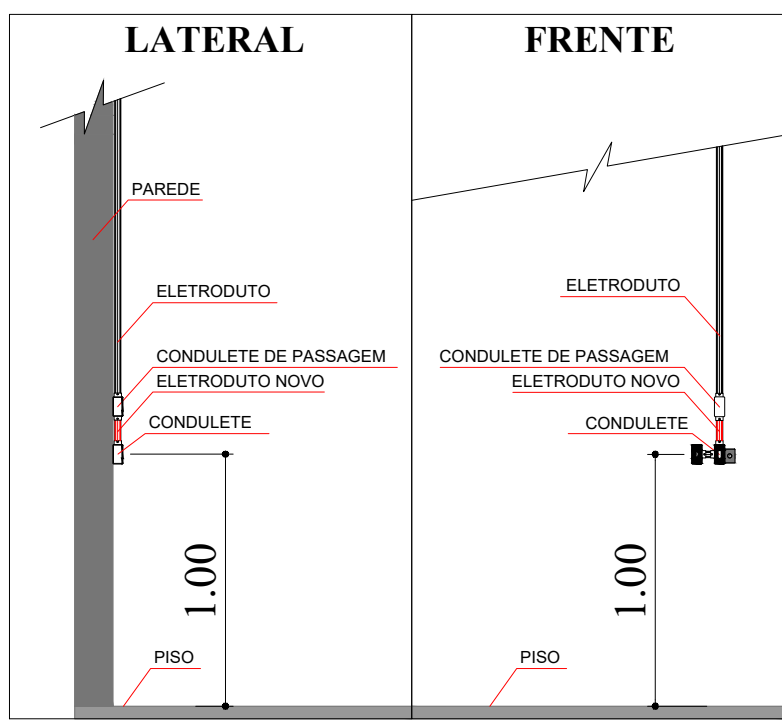
INTERRUPTOR / TOMADA AJUSTADOS
