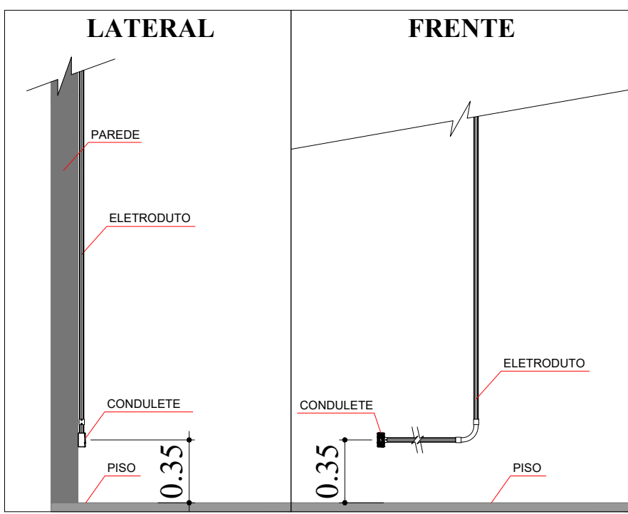
TOMADA EXISTENTE
