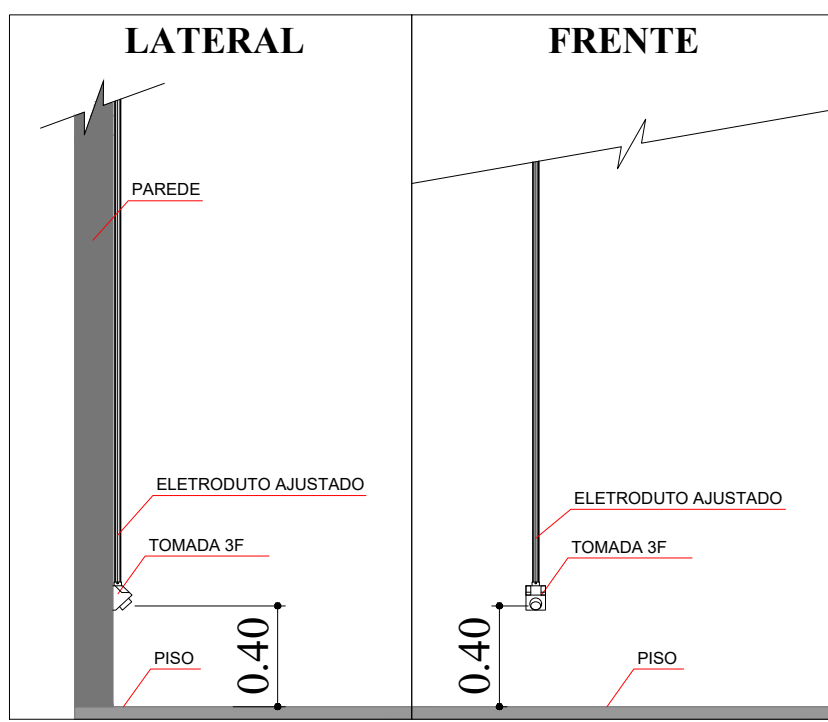
TOMADA AJUSTADA
