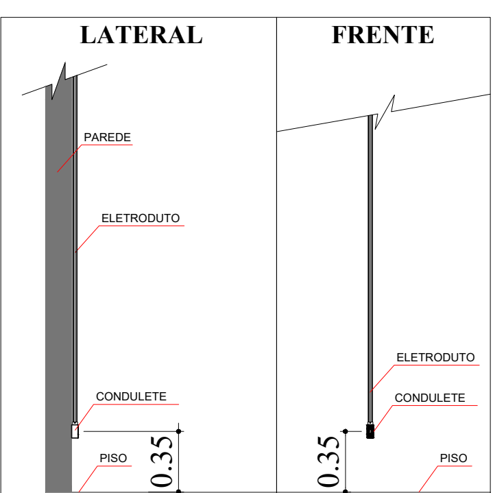
TOMADA EXISTENTE
