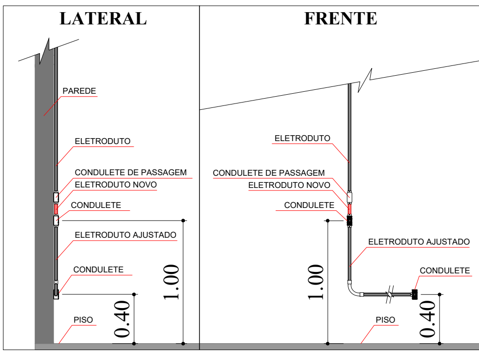
TOMADAS AJUSTADAS
