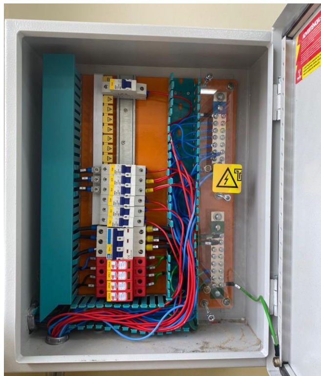
Registro Fotográfico nº 32 – Quadro elétrico da sala 206-B (LICC 2)
