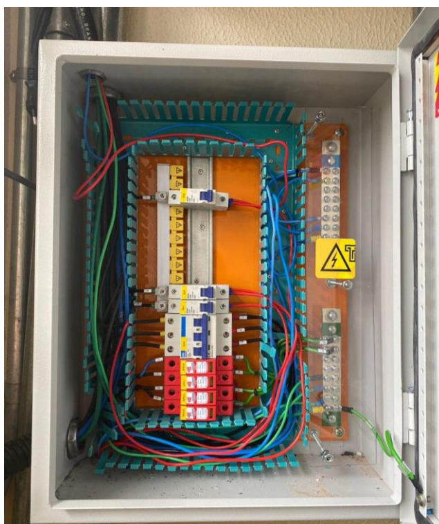
Registro Fotográfico nº 28 – Quadro elétrico da sala 206-A (LICC 1)
