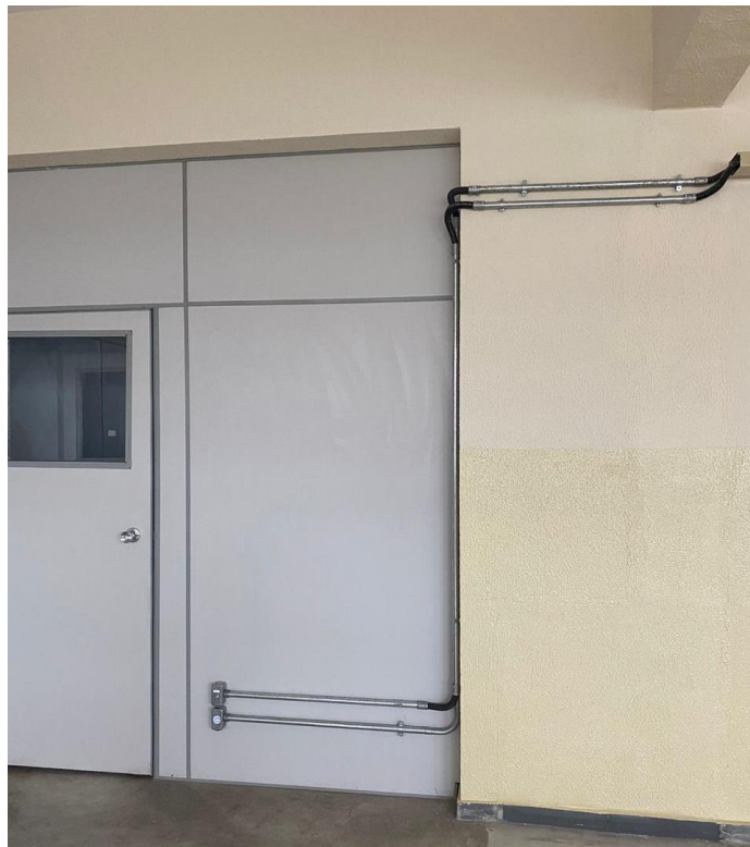
Registro Fotográfico nº 36 – Finalização das instalações elétricas e de cabeamento da sala de aula 201
