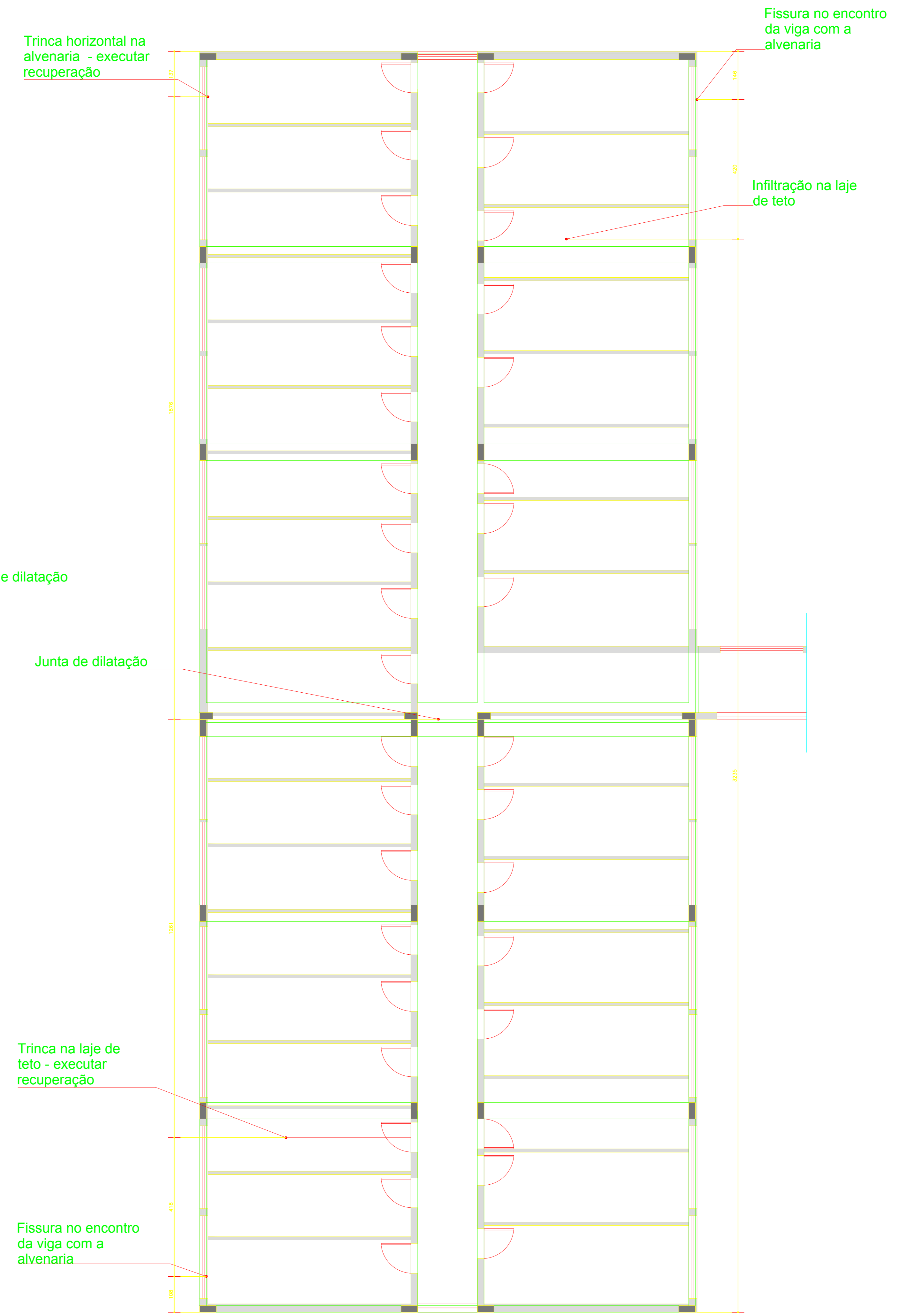
PLANTA - BLOCO A - NÍVEL +7,00 Escala 1:100
